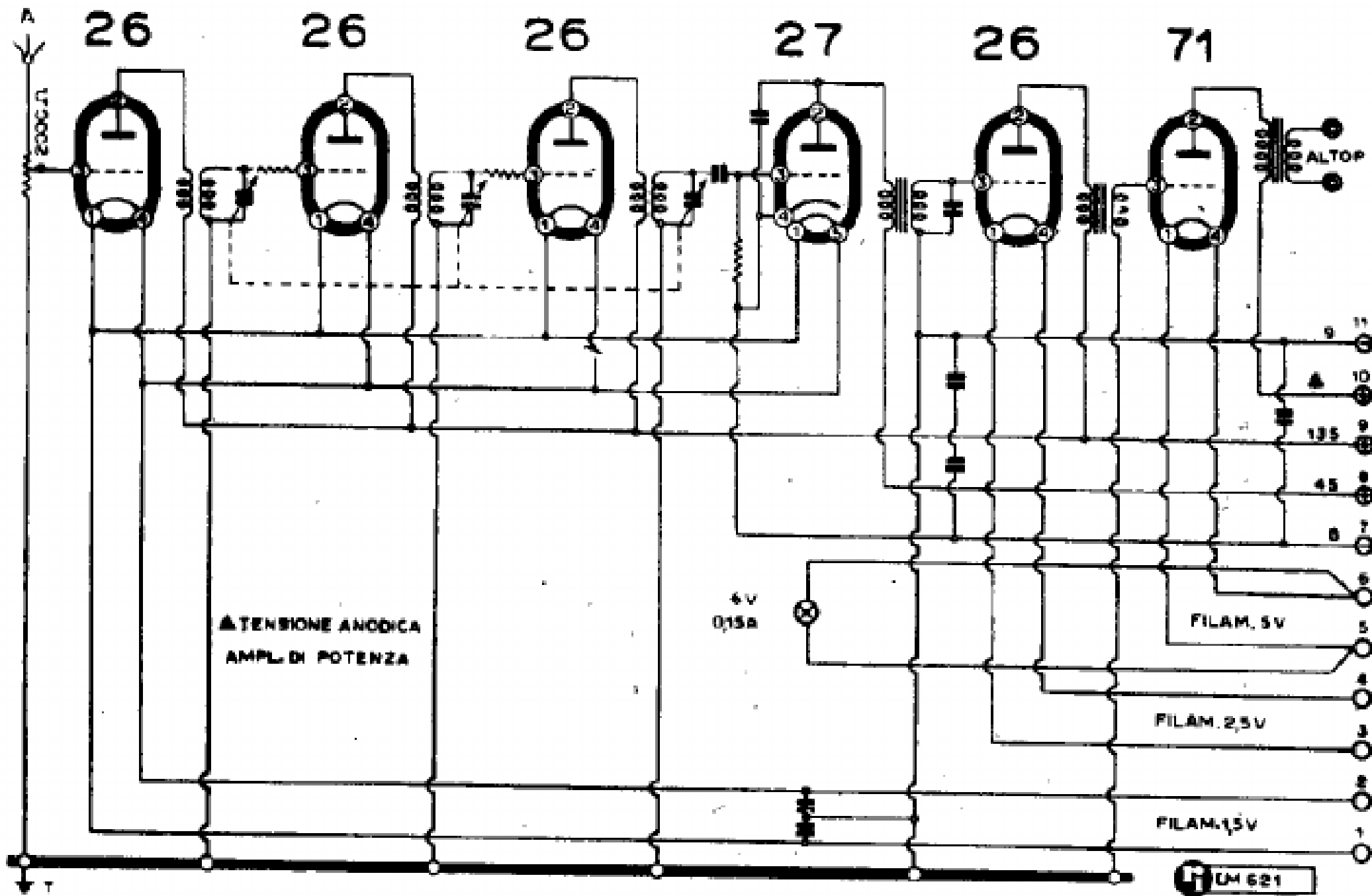
COMPAGNIA GENERALE DI ELETTRICITA' - MOD. « RADIOLA 17 »
